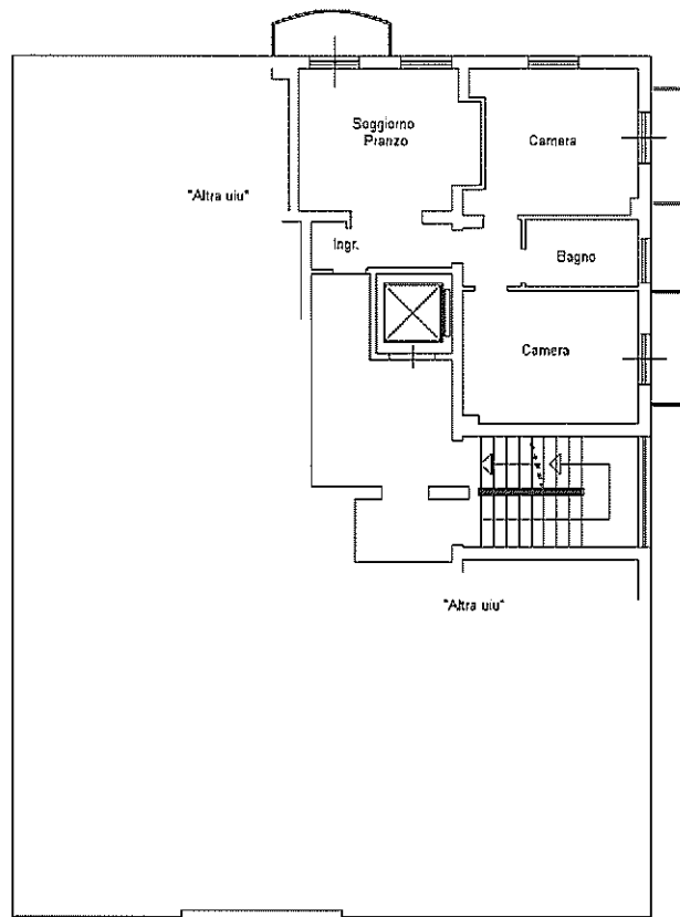
Piano Secondo H= 2.90
