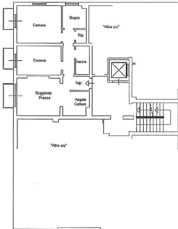
Piano Primo H=2.90
