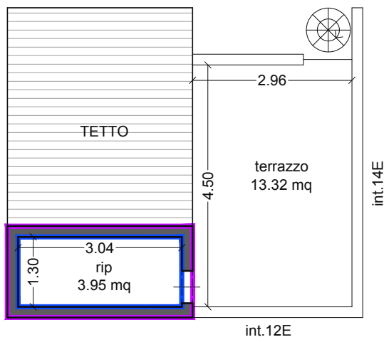
PIANTA COPERTURA
